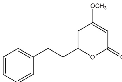
Dihydrokavain
