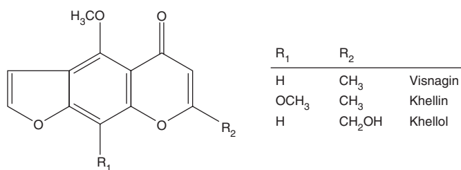
Furanochromones
