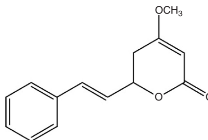
Kavain
