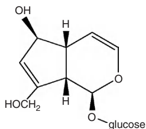
Aucubin
