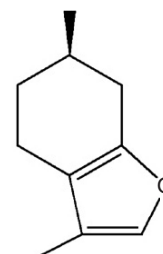
Menthofuran
