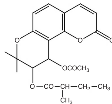
Visnadin
