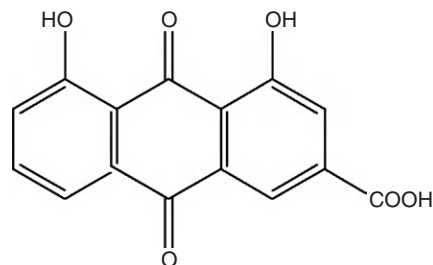
Rhein
