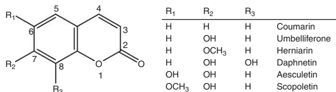
Simple coumarins
