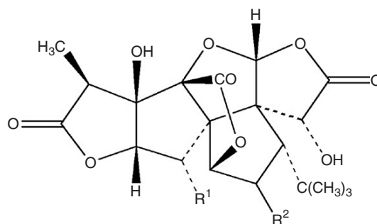
Ginkgolides
